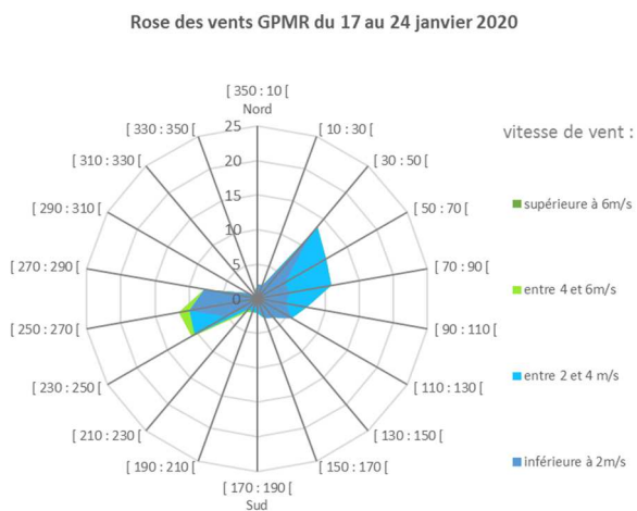
Figure 29 : Rose des vents du 17 au 24/01/20 (à gauche) et localisation des sites concernés (à droite) – source : Atmo Normandie
