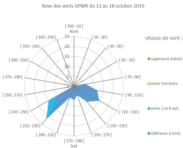
Figure 32 : Rose des vents du 11/10 au 18/10/19 (à gauche) et localisation des sites concernés (à droite) – source : Atmo Normandie
