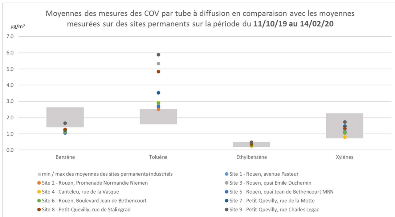
Figure 25 : Moyennes des mesures de COV par tube à diffusion en comparaison avec les moyennes mesurées sur des sites permanents sur la période du 11/10/19 au 14/02/20 – source : Atmo Normandie
