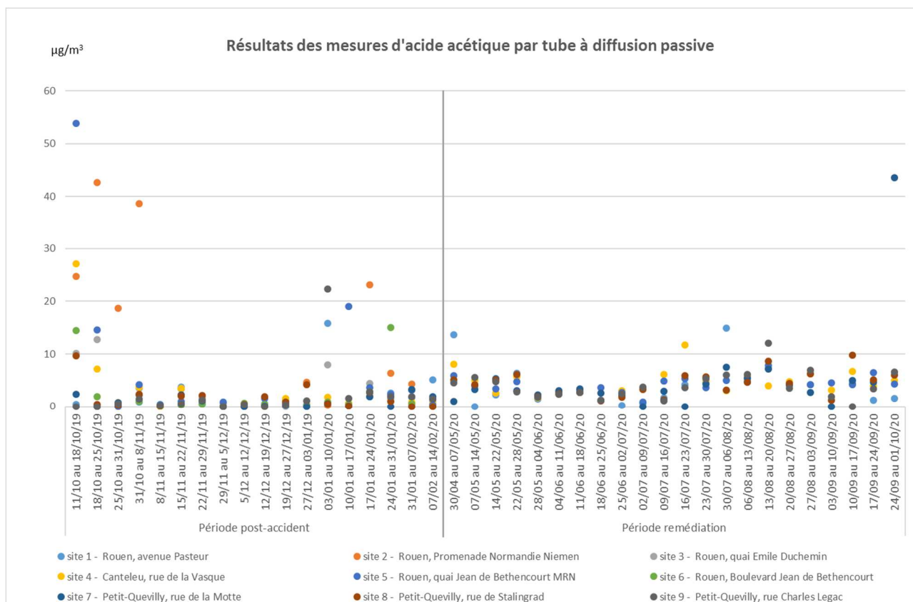
Figure 31 : Concentrations en acide acétique par campagne de mesure et par site – source : Atmo Normandie
