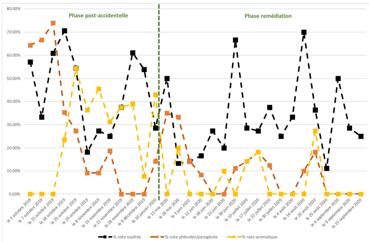
Figure 23 : Evolution des 3 principales familles repérées lors des tournées olfactives effectuées par les Nez d'Atmo Normandie (phase post-accidentelle du 03/10/19 au 10/01/20 et phase remédiation du 13/05/20 au 15/09/20) – source : Atmo Normandie
