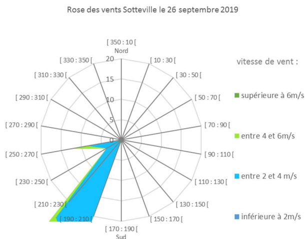
Figure 6 : Rose des vents du 26/09/19 - Source : Atmo Normandie
