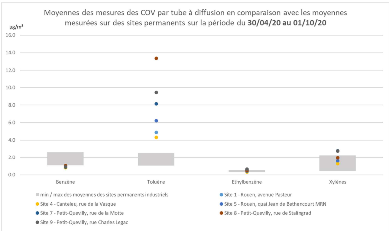
Figure 26 : Moyennes des mesures de COV par tube à diffusion en comparaison avec les moyennes mesurées sur des sites permanents sur la période du 30/04/20 au 01/10/20 – source : Atmo Normandie
