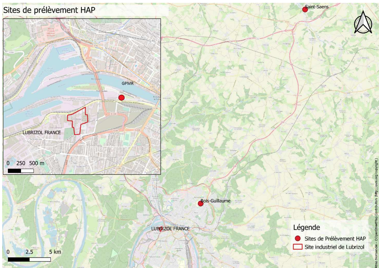
Figure 14 : Localisation des sites de prélèvements de HAP – source : Atmo Normandie
