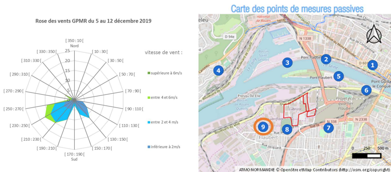
Figure 28 : Rose des vents du 5 au 12/12/19 (à gauche) et localisation des sites concernés (à droite) – source : Atmo Normandie
