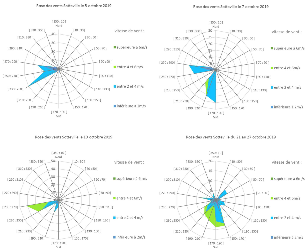
Figure 10 : Roses des vents des 5, 7, 10 et du 21 au 27/10/19 - Source : Atmo Normandie
