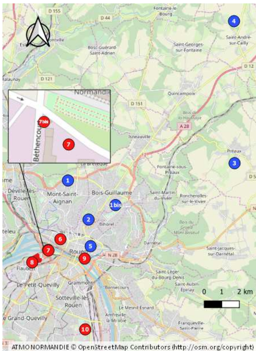
Figure 16 : Localisation des sites de mesure des retombées atmosphériques – source : Atmo Normandie
