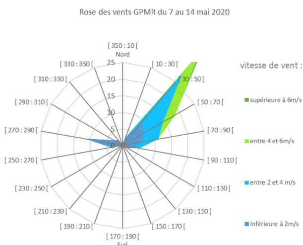
Figure 30 : Rose des vents du 7 au 14/05/20 (à gauche) et localisation des sites concernés (à droite) – source : Atmo Normandie
