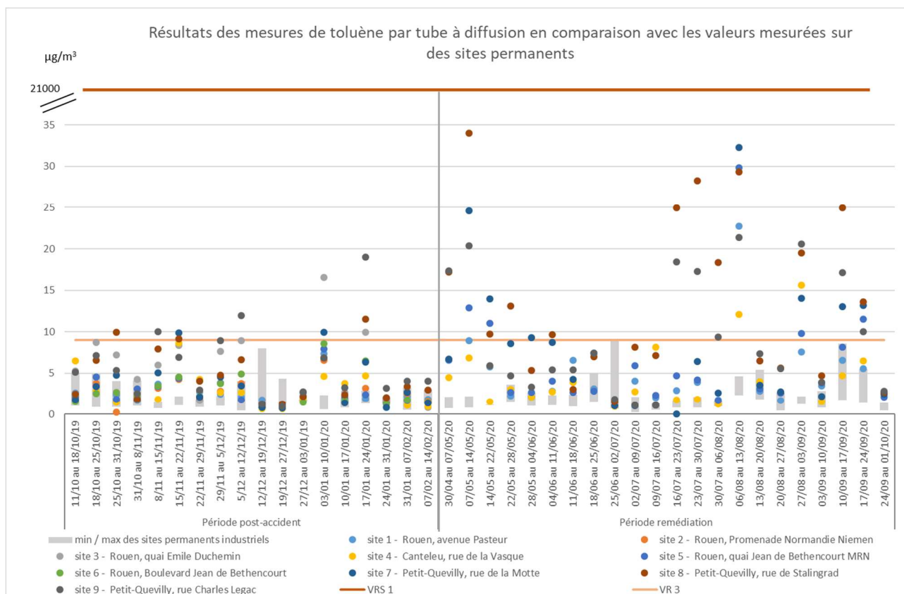
Figure 27 : Concentrations en toluène par campagne de mesure et par site, comparaison avec des valeurs de référence sanitaire et mesurées sur des sites permanents – source : Atmo Normandie
