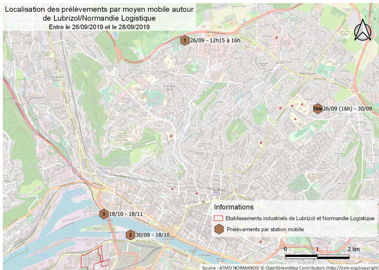
Figure 13 : Evolution chronologique de la localisation du moyen mobile de mesures automatiques en continu – source : Atmo Normandie
