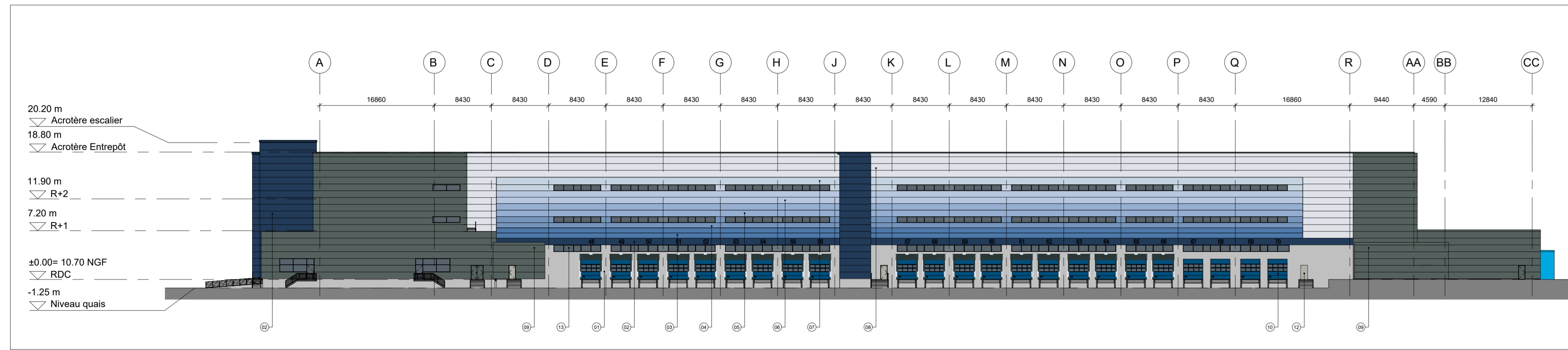
Façade Sud-Est Echelle: 1/400
