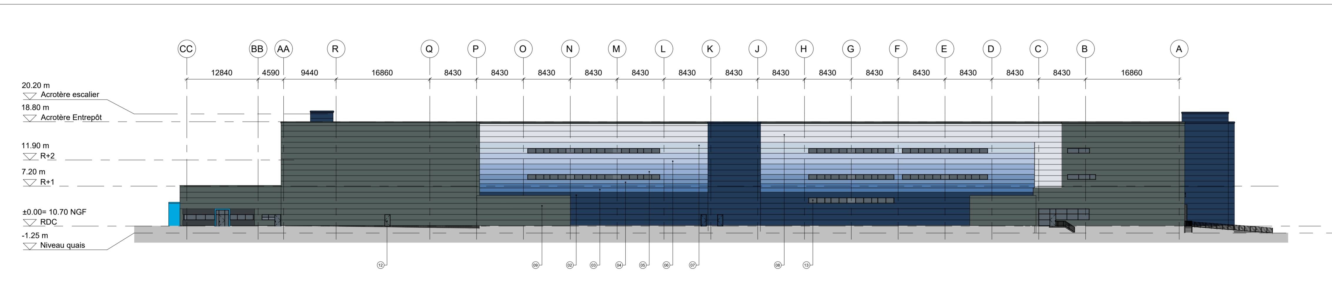
Façade Nord-Ouest Echelle: 1/400
