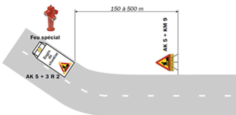
Cas des contrôles réalisés sur des chaussées sous circulation en l'absence de visibilité.
