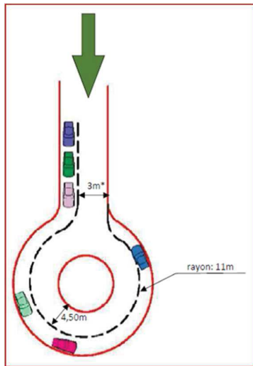
Aire de retournement circulaire
